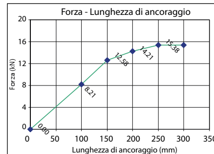
Fig. 1. Grafico Forza di delaminazione lunghezza di ancoraggio per muratura in mattoni in argilla.
